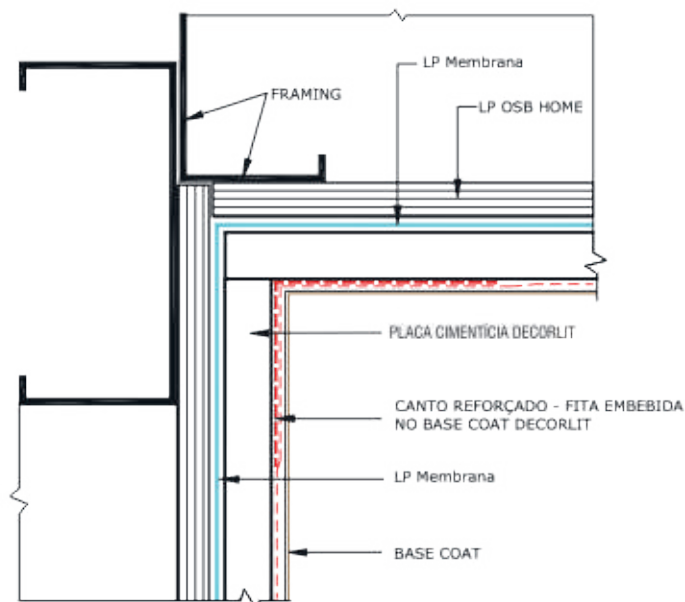
DECORLIT D1.01 CANTO INTERNO
