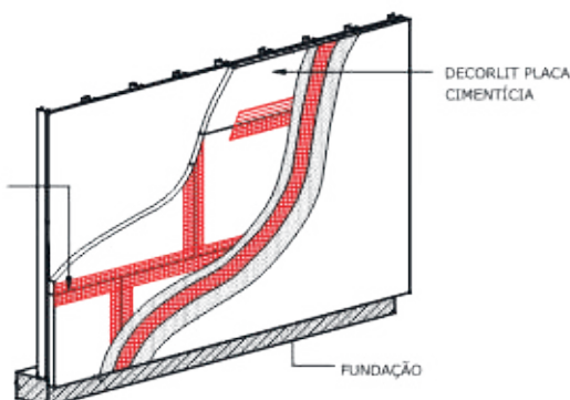
ADITIVO FLEX + BASE COAT + FITA TELADA DE 100 MM DECORLIT
