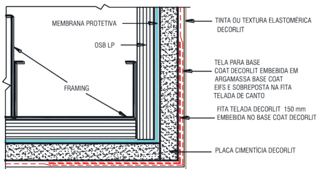
DECORLIT D1.02 CANTO EXTERNO
