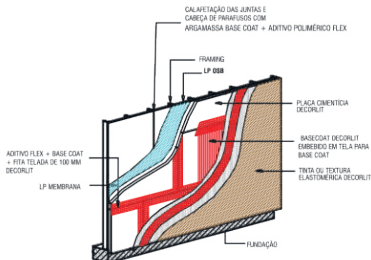
D2.01 APLICAÇÃO DE SISTEMA BASE COAT EM WOOD/STEEL FRAME
