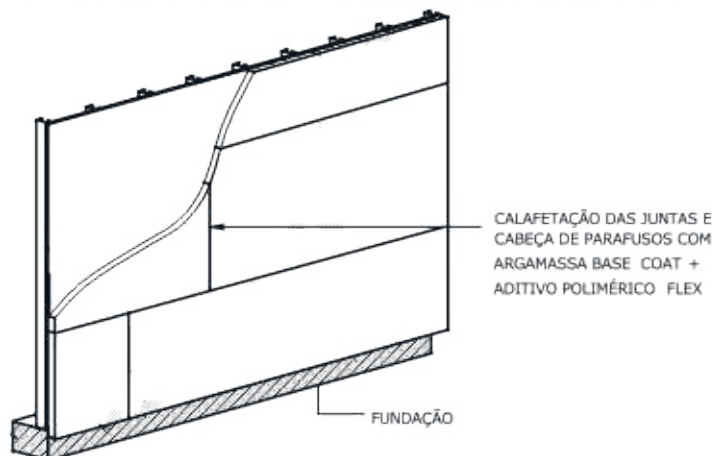
D2.01 APLICAÇÃO DE SISTEMA BASE COAT EM WOOD/STEEL FRAME
