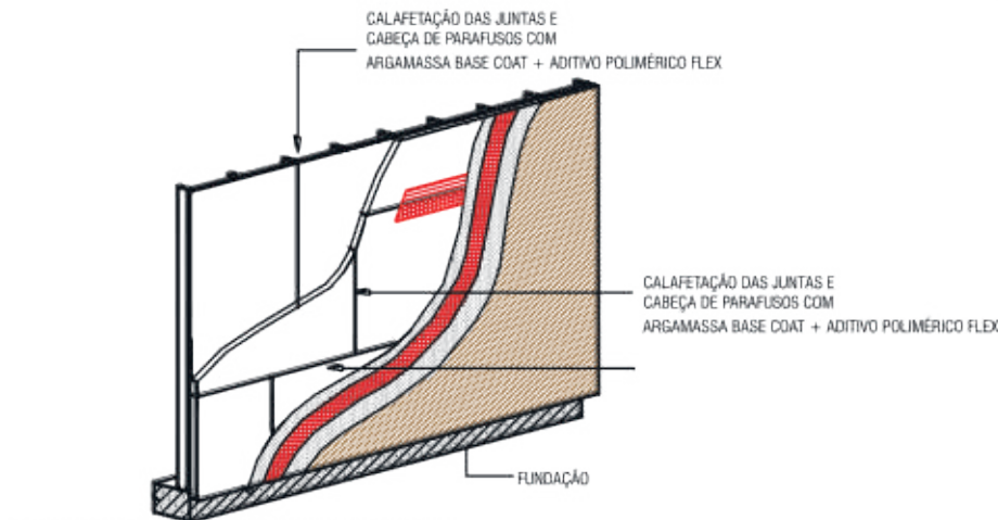
D2.01 APLICAÇÃO DE SISTEMA BASE COAT EM WOOD/STEEL FRAME
